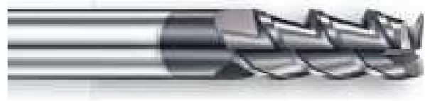
Sarkos 3 élű normál hosszúságú TiAlN bevonatos marók 55HRC keménységig
